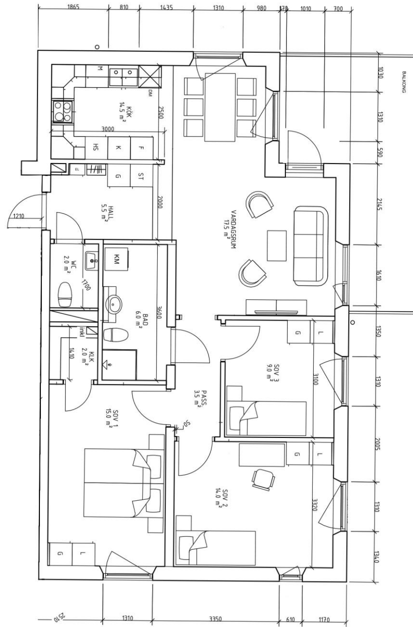
Planlösning skala 1:100
