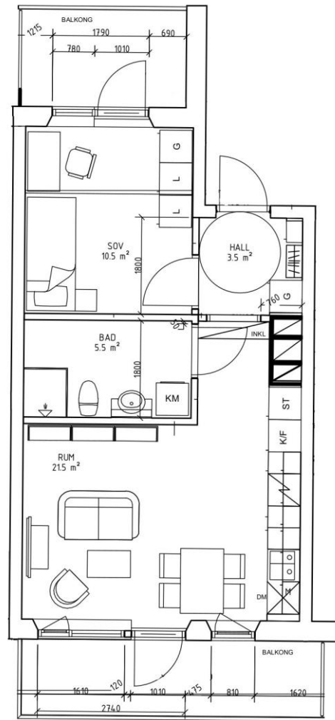
Planlösning skala 1:100
