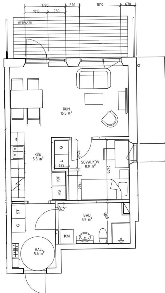
Planlösning skala 1:100
