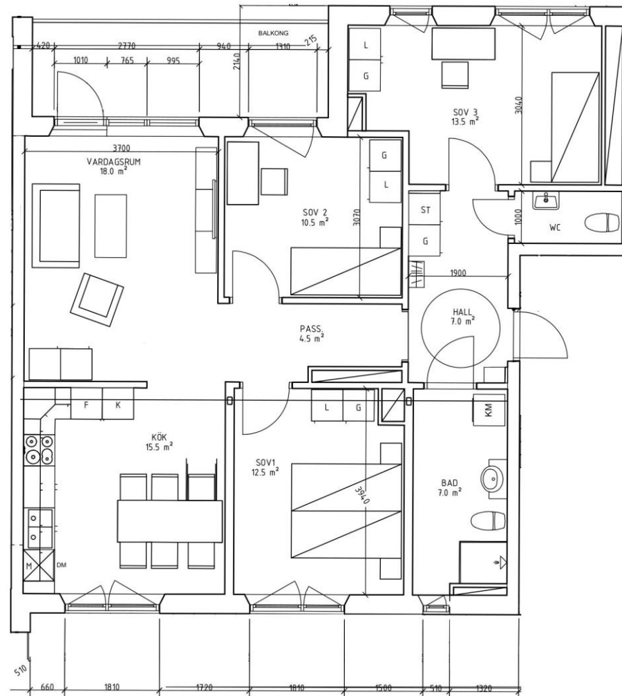
Planlösning skala 1:100
