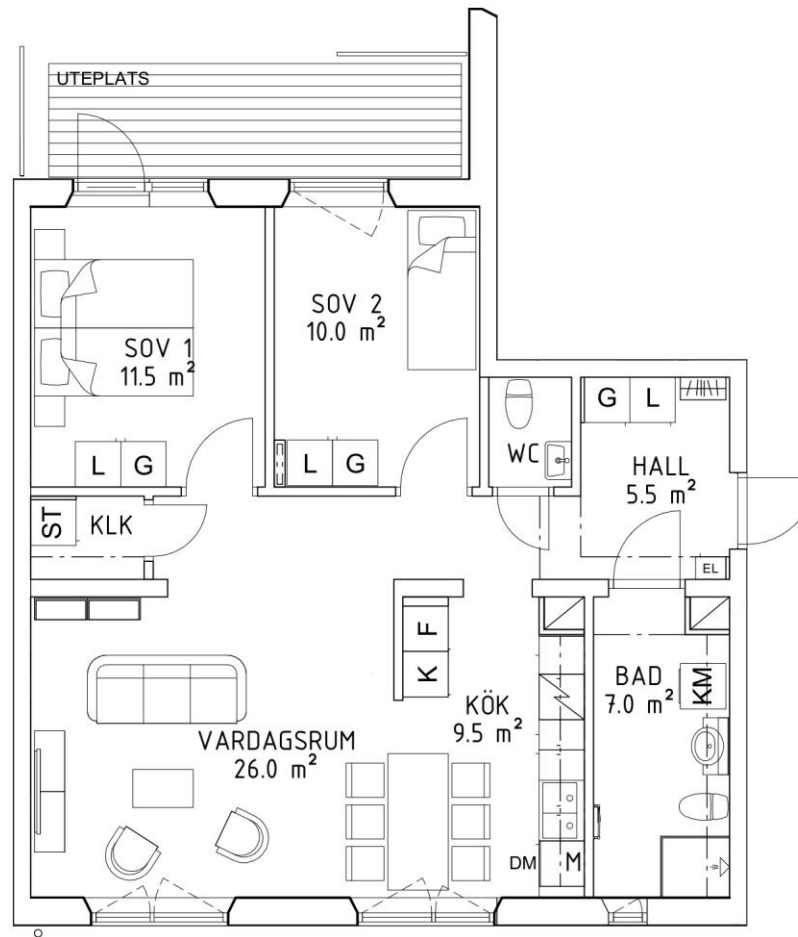
Planlösning skala 1:100
