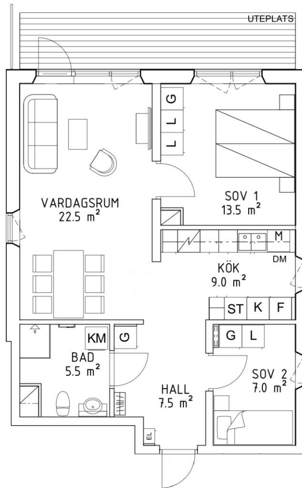
Planlösning skala 1:100
