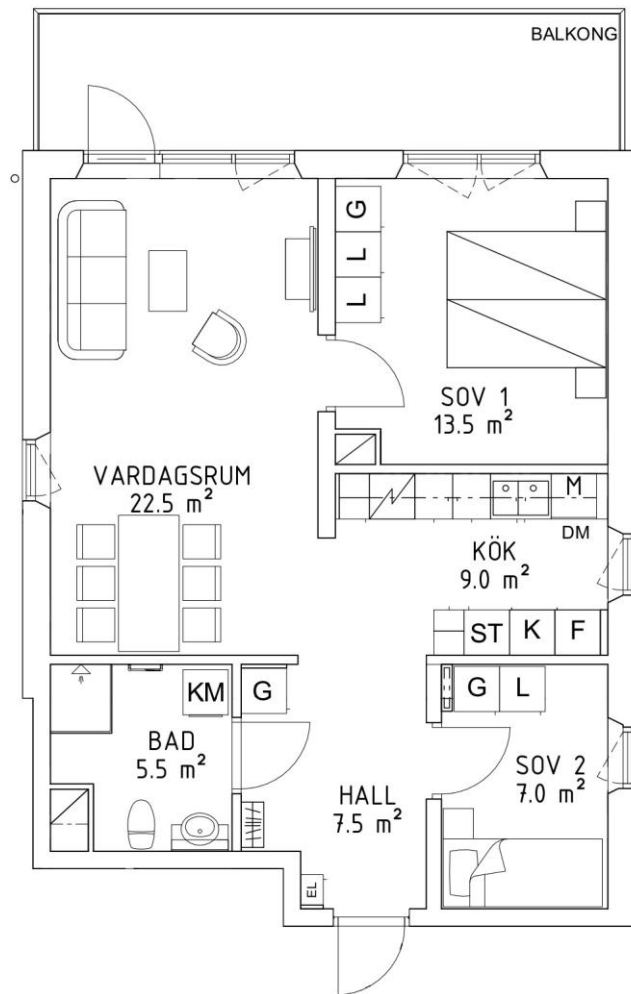
Planlösning skala 1:100
