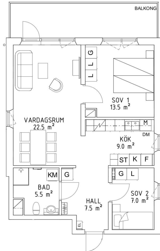
Planlösning skala 1:100
