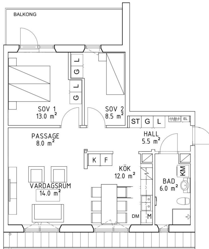
Planlösning skala 1:100
