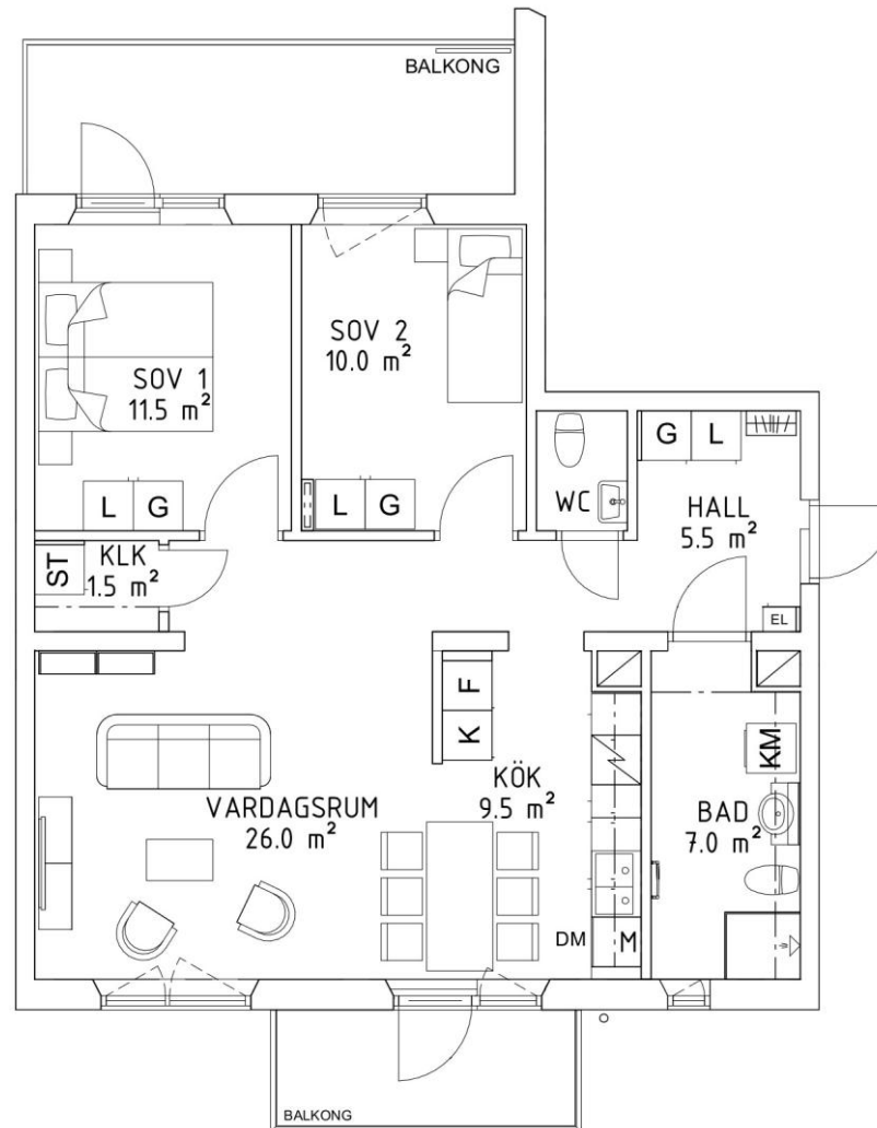
Planlösning skala 1:100
