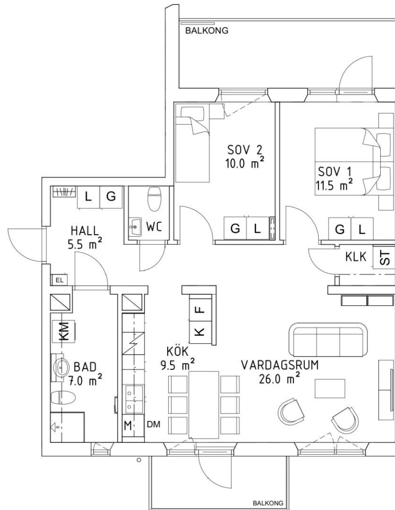
Planlösning skala 1:100
