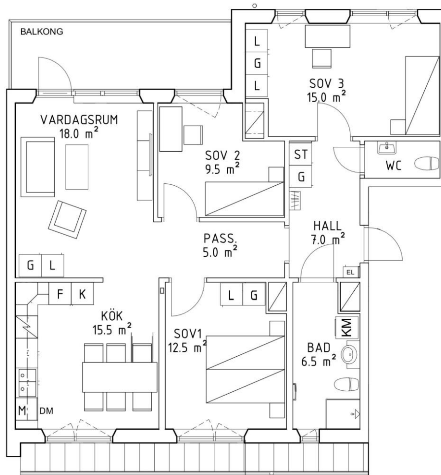
Planlösning skala 1:100
