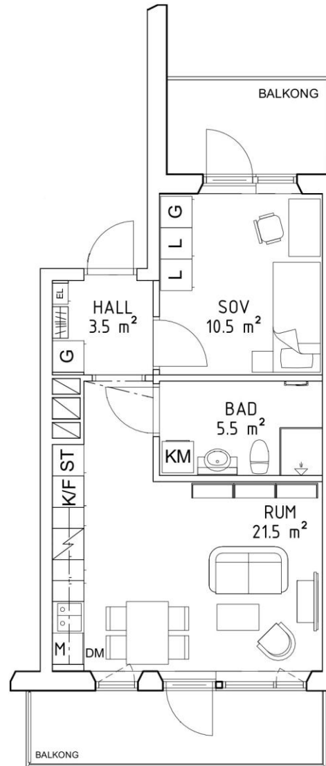
Planlösning skala 1:100
