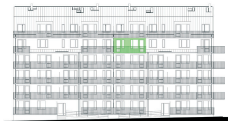
Fasad mot gård, väster
