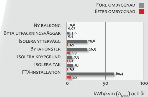
Energibesparingen av fjärrvärme för uppvärmning visat per åtgärd.
